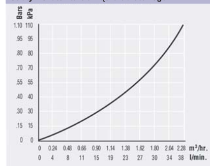
Straty wskutek tarcia złącza obrotowego
